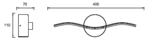
Dimension(mm)
