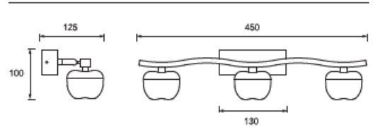
Dimension(mm)
